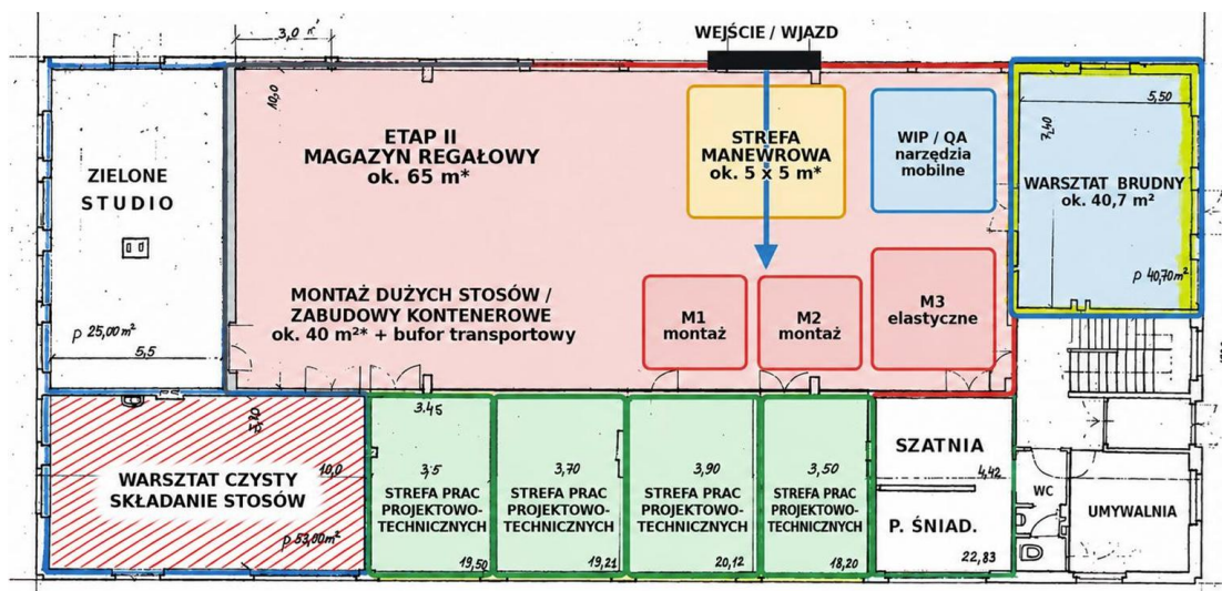
Rys. 1. Schemat funkcjonalnego podziału i zagospodarowania powierzchni produkcyjno-montażowej ***.
